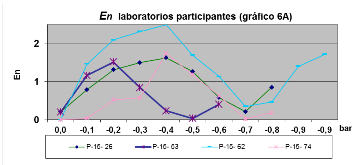
Gráfico 6A. Curvas del error normalizado |E_n| > 1.0 Resultado NO satisfactorio
