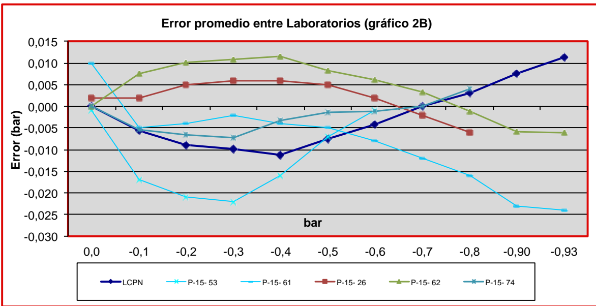
Gráfico 2B. Curvas de error, E , de los laboratorios con menor concordancia.
