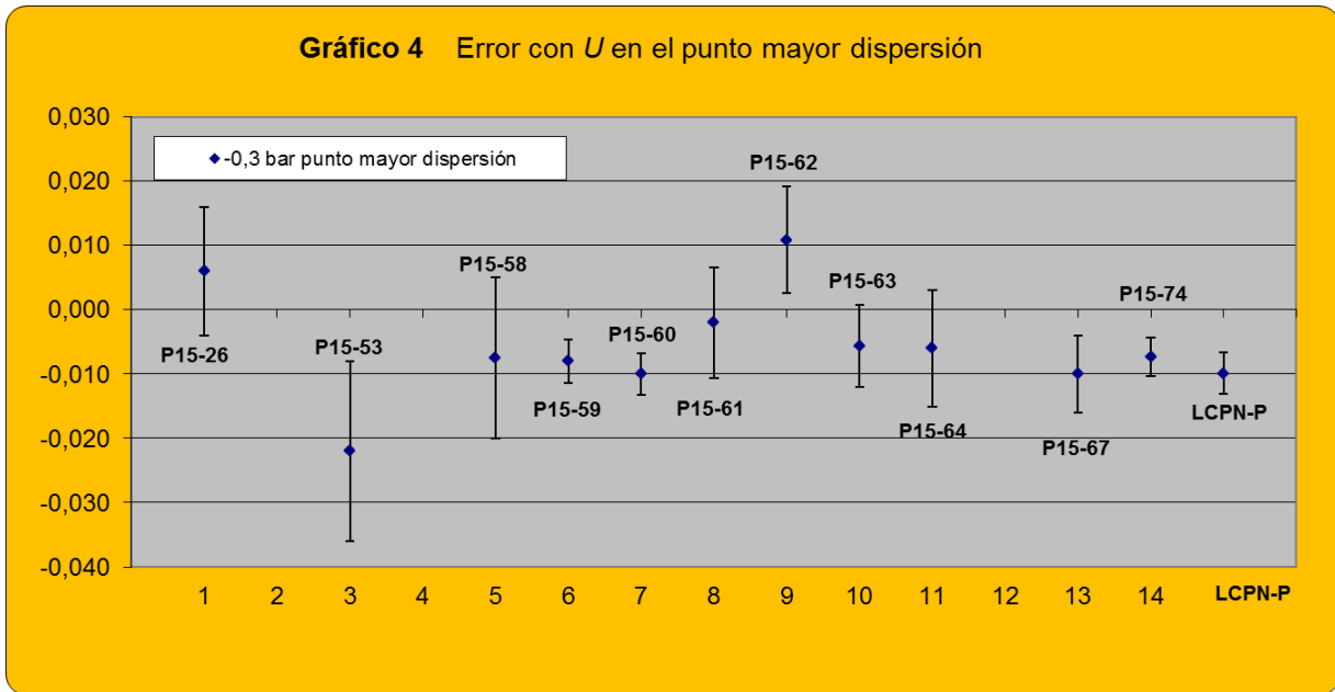
Gráfico 4. Datos de error promedio E , con incertidumbre expandida, U , en el punto de medición con mayor dispersión
