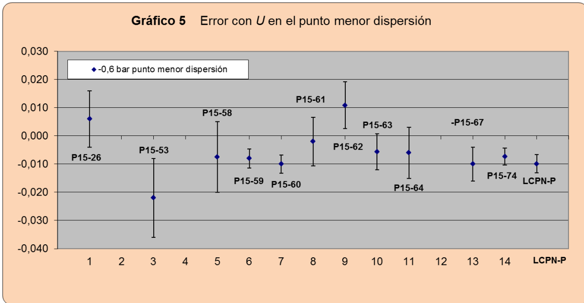
Gráfico 5. Datos de error promedio E , con incertidumbre expandida, U , en el punto de medición con menor dispersión.
