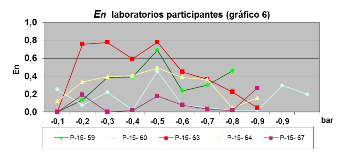
Gráfico 6. Curvas del error normalizado |E_n| \leq 1.0 Resultado satisfactorio
