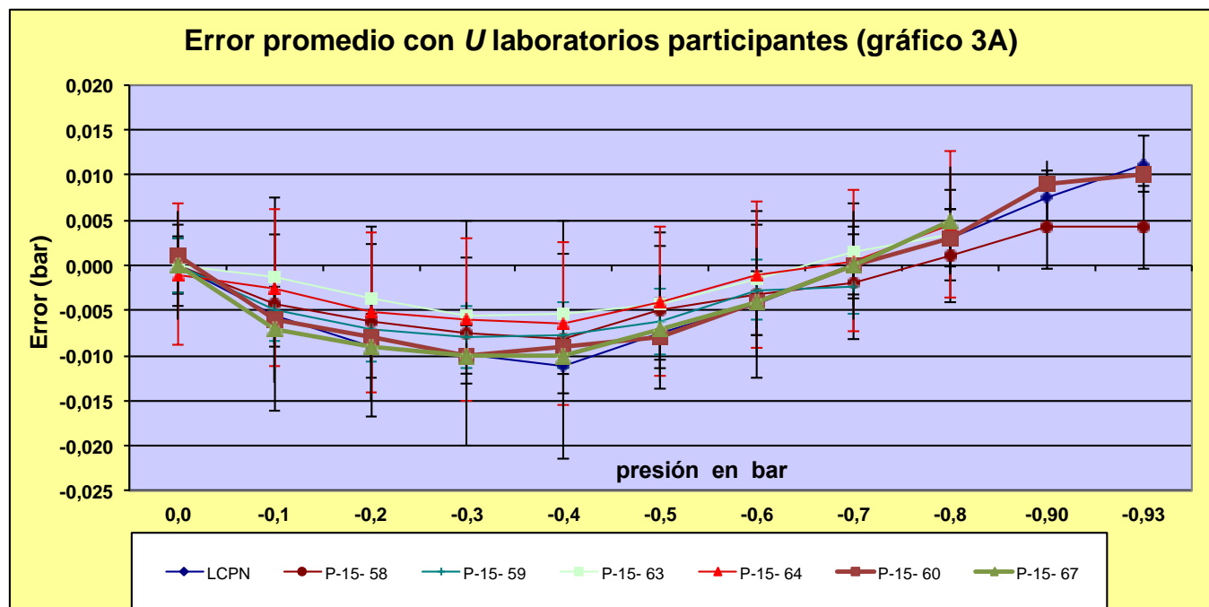
Gráfico 3A. Datos de error promedio, E , con incertidumbre expandida, U , Laboratorios con mejor concordancia.
