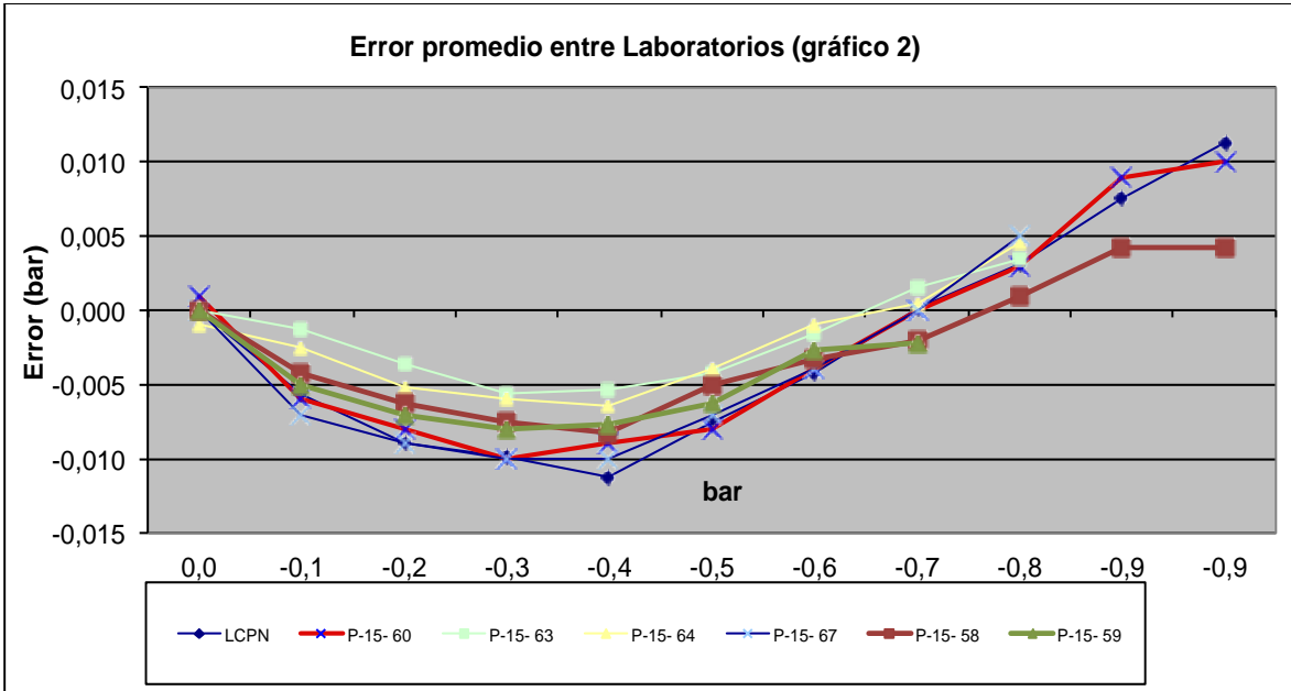
Gráfico 2. Curvas de error, E , de los laboratorios con mejor concordancia.
