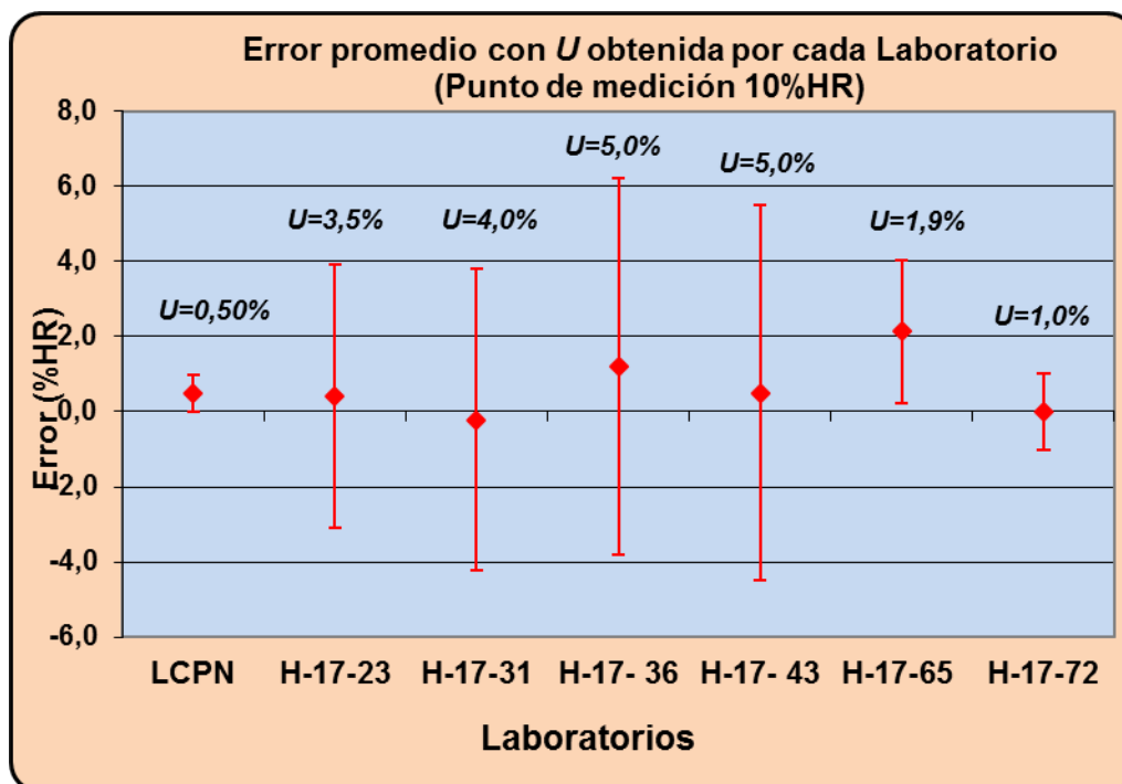
Gráfico 6. Error promedio entre laboratorios con incertidumbre (10% HR).
