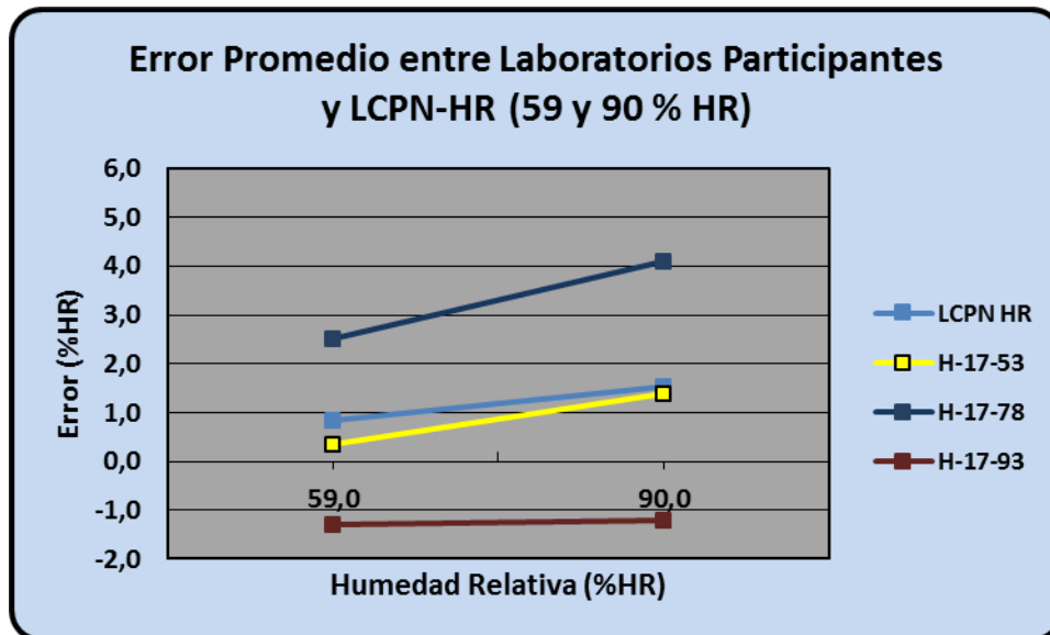
Grafico 5. Error promedio entre laboratorios en 59 y 90 % HR.
