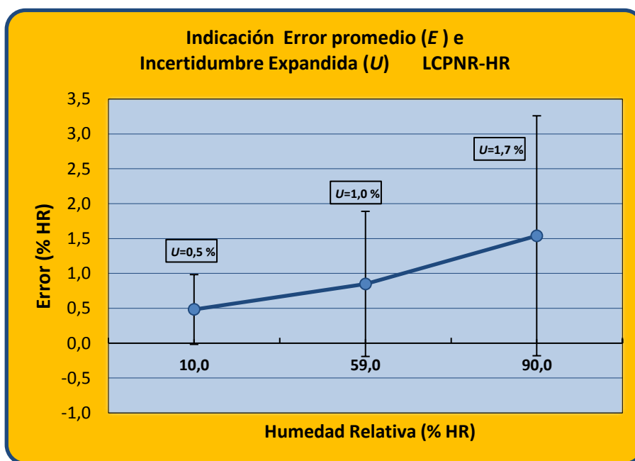
Gráfico 2. Error promedio., E , e incertidumbre expandida, U ( k=2 , 95%). Laboratorio LCPNR-HR.
