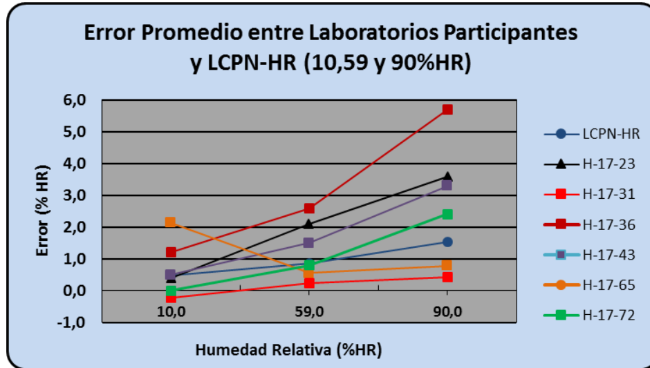
Grafico 4. Error promedio entre laboratorios en 10,59 y 90 % HR.
