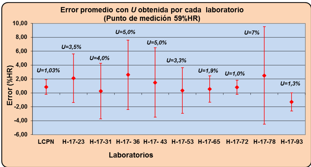
Gráfico 7. Error promedio entre laboratorios con incertidumbre (59%HR).
