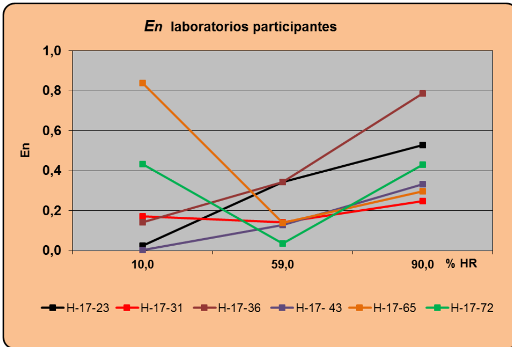
Gráfico 11. Errores normalizados de todos los laboratorios.
