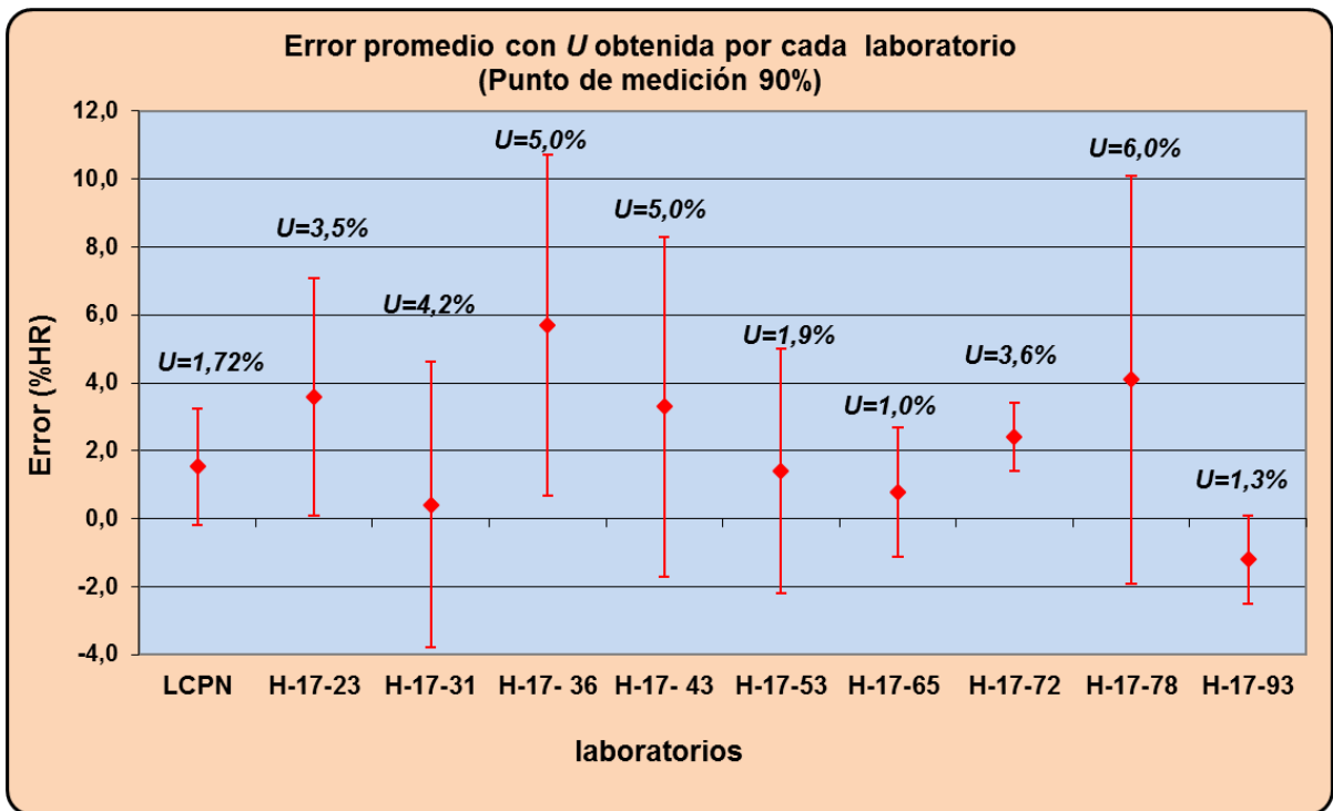
Gráfico 8. Error promedio entre laboratorios con incertidumbre (90%HR).
