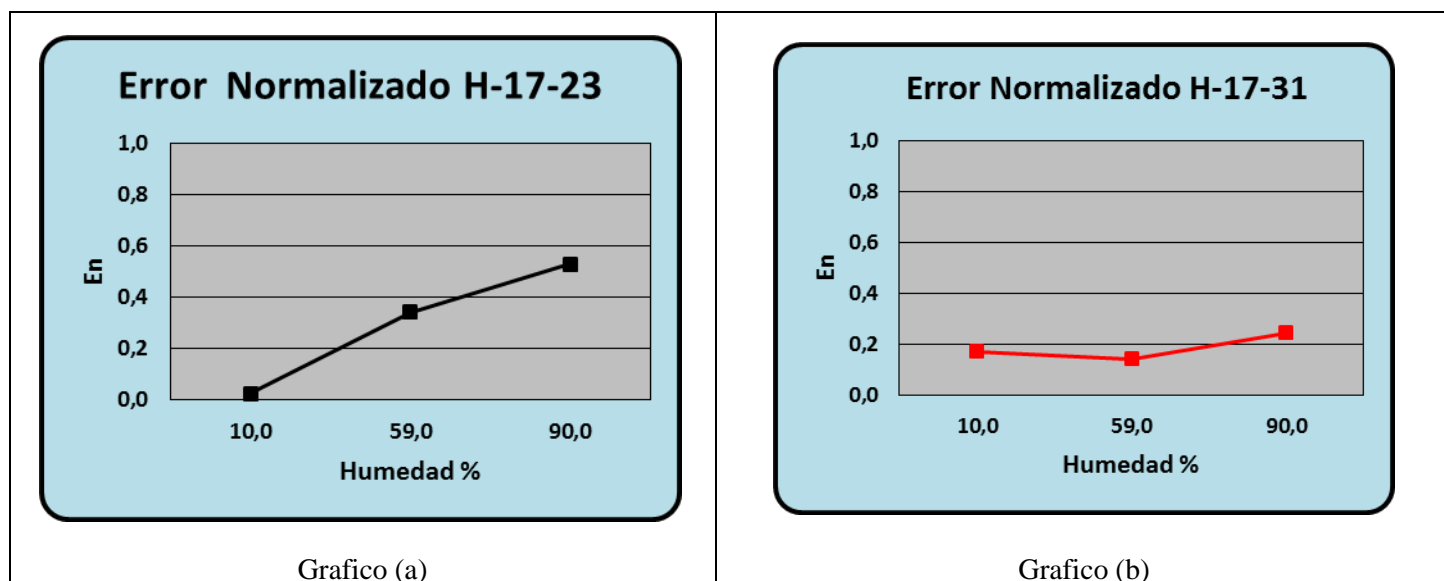
Gráfico 9. Errores normalizados individuales de cada laboratorio participante.
