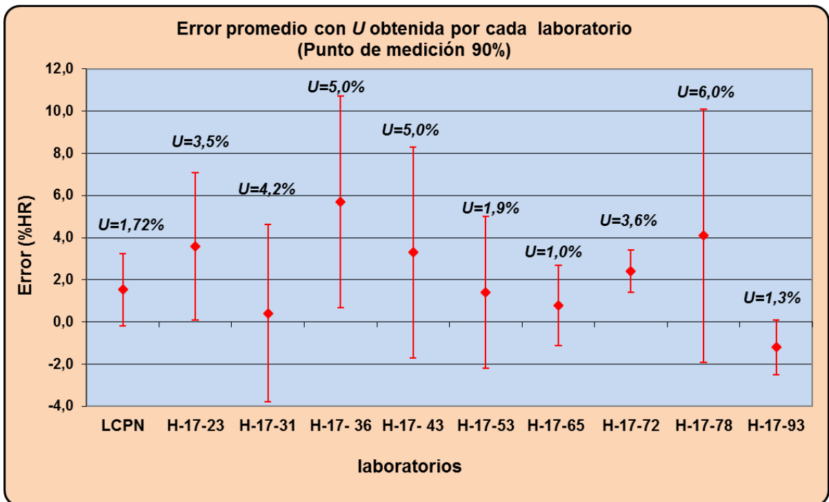
Gráfico 8. Error promedio entre laboratorios con incertidumbre (90%HR).
