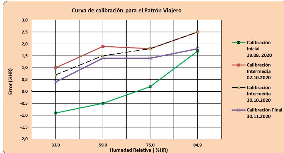
Gráfico 1. Error de medición encontrado para el patrón viajero en las calibraciones realizadas por el LCPNR-HR de ENAER.
