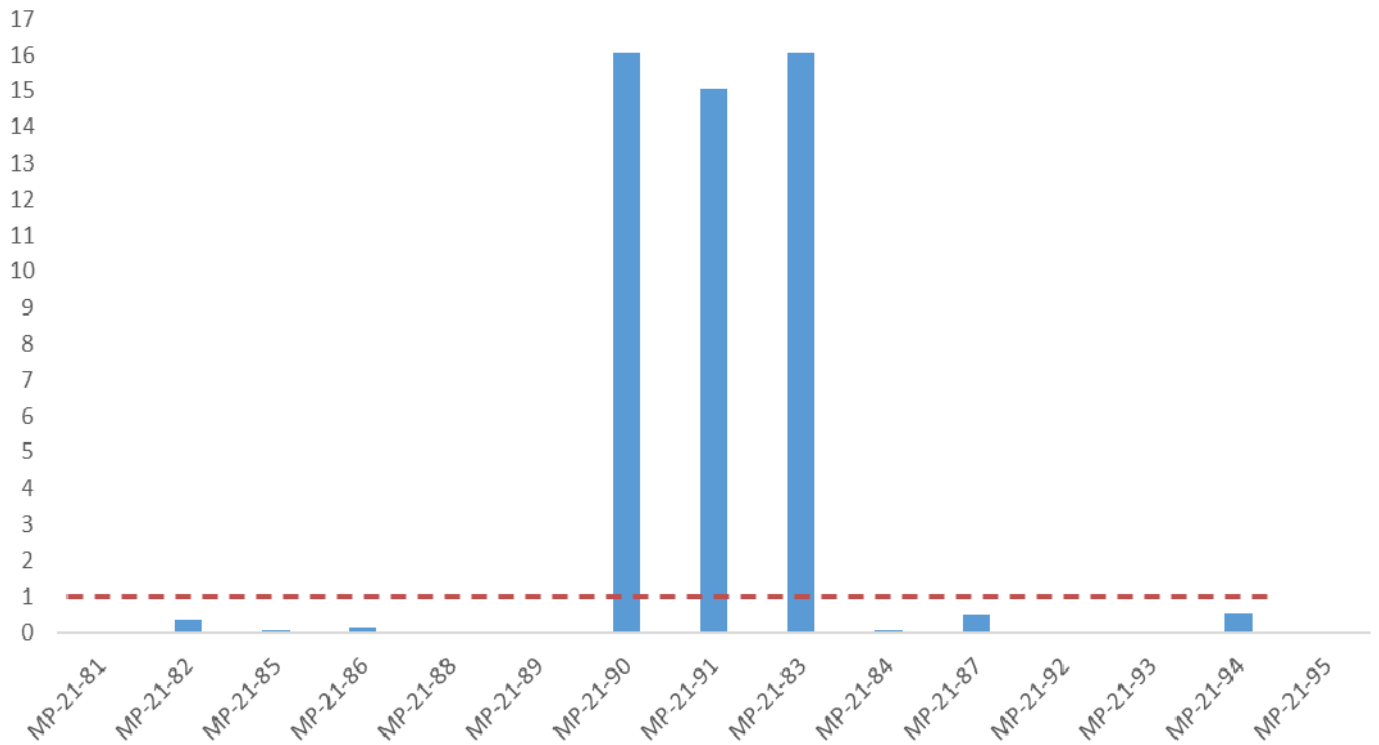
Error normalizado en pesa de valor nominal 1 g
