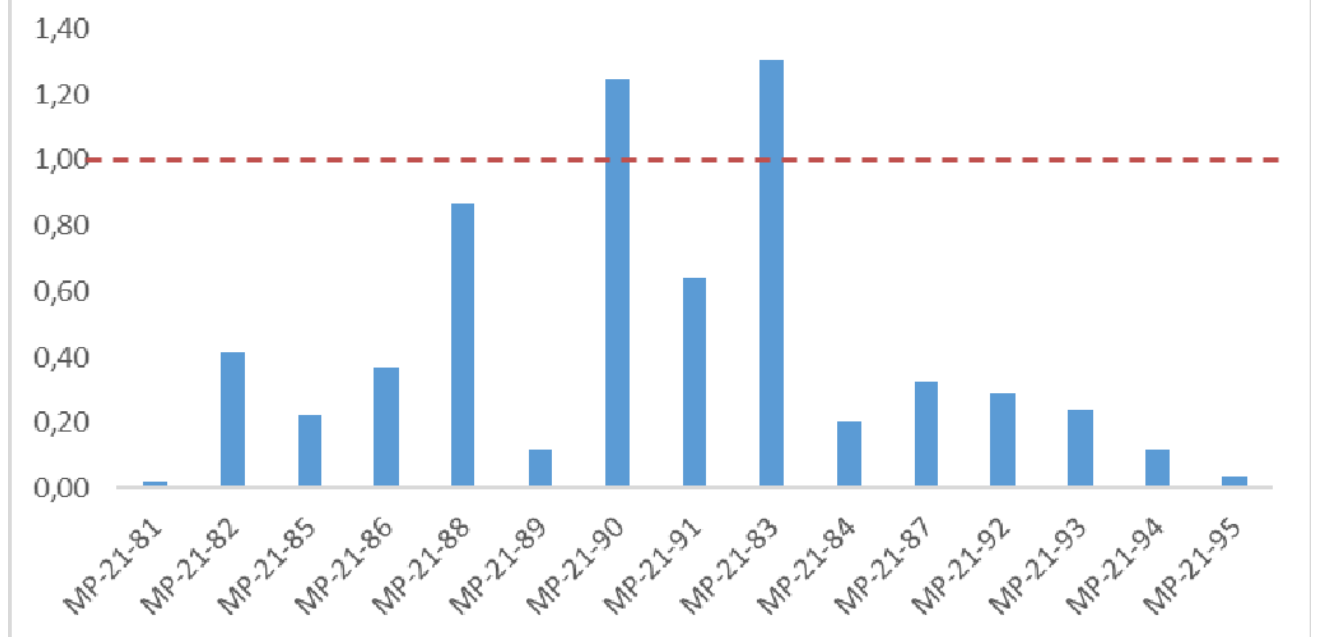
Error normalizado en en pesa de valor nominal 5 kg
