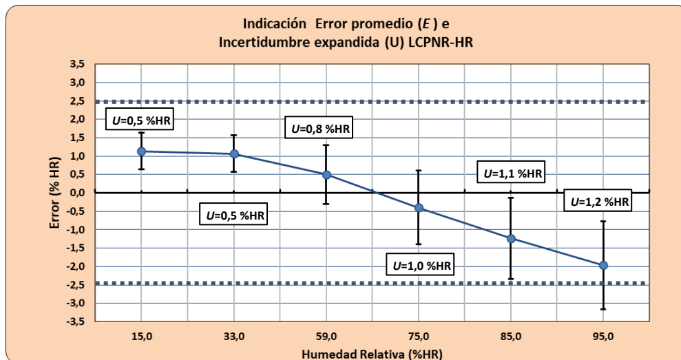
Gráfico 2. Error promedio, E, e incertidumbre expandida, U (k=2, 95%) obtenida por el LCPNR-HR ENAER. (Las líneas de puntos corresponden a la exactitud del instrumento) (La incertidumbre en este gráfico es la máxima entre las 3 calibraciones).
