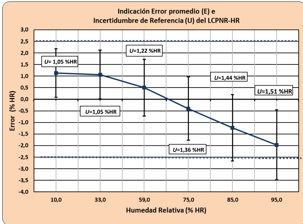
Gráfico 3. Error promedio, E , e incertidumbre del laboratorio de referencia, U ( k=2 , 95%), con consideración adicional por deriva del patrón viajero. (Las líneas de puntos corresponden a la exactitud del instrumento).
