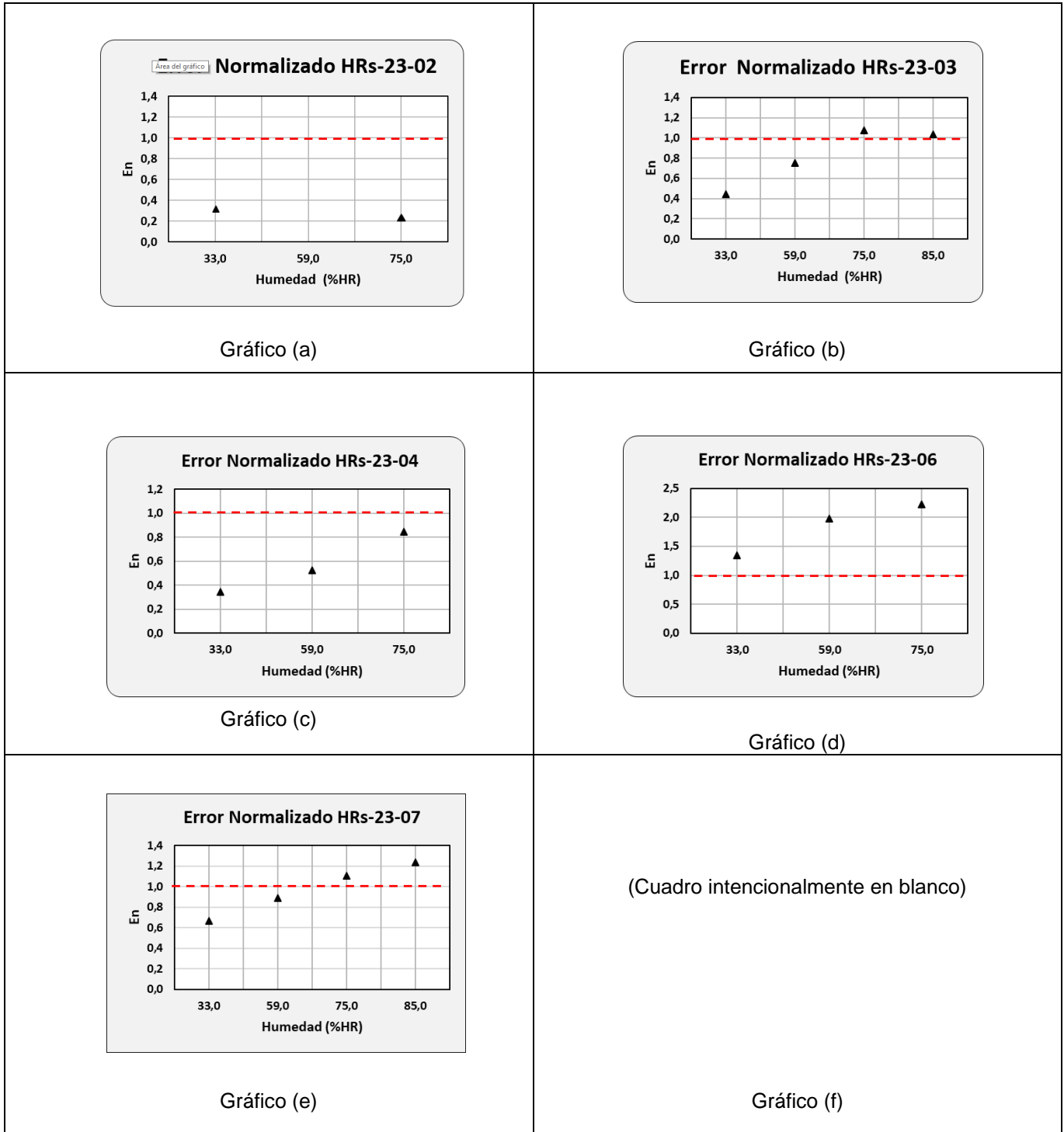
Gráfico 12. Errores normalizados individuales de cada laboratorio participante.
