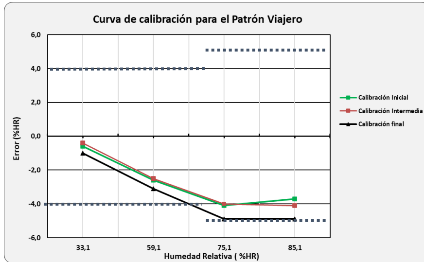
Gráfico 1. Error de medición encontrado para el patrón viajero en las calibraciones realizadas por el LCPNR-HR de ENAER (Las líneas de puntos corresponden a la exactitud del instrumento).
