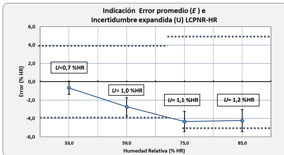
Gráfico 2. Error promedio, E , e incertidumbre expandida, U ( k=2 , 95%) obtenida por el LCPNR-HR ENAER.
