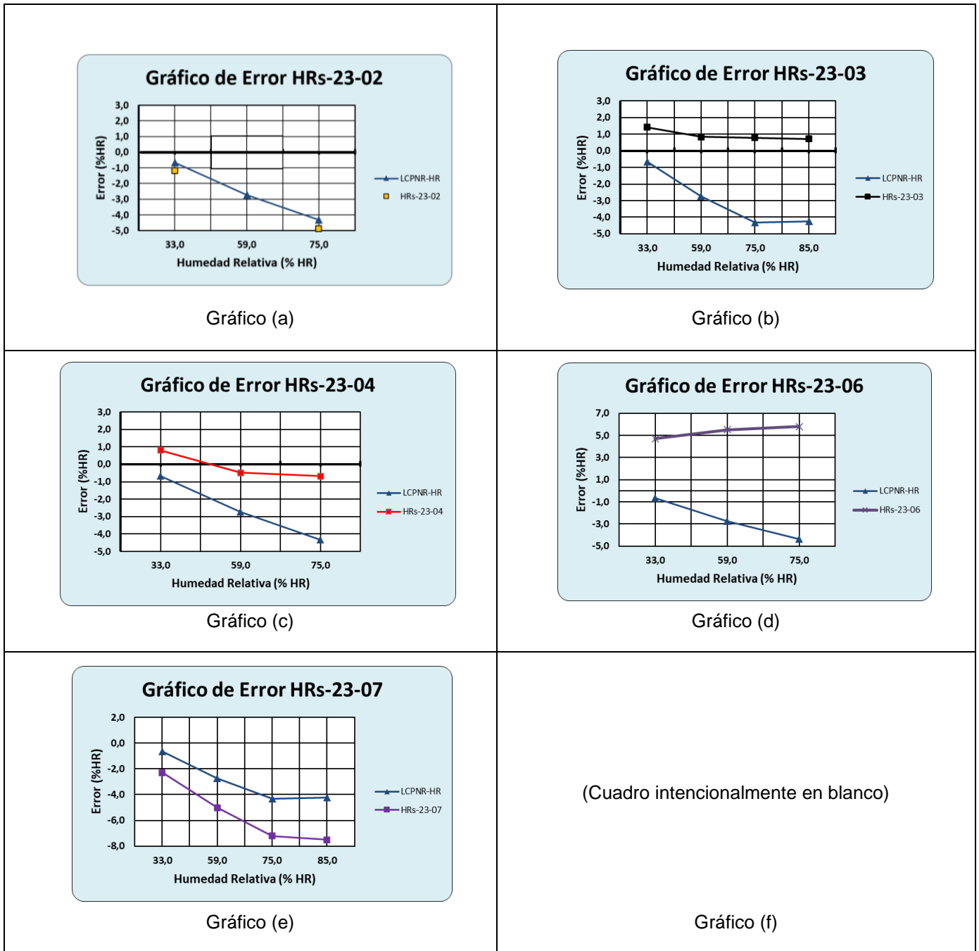
Gráfico 4. Error Individual de cada participante con respecto a LCPNR-HR de ENAER.
