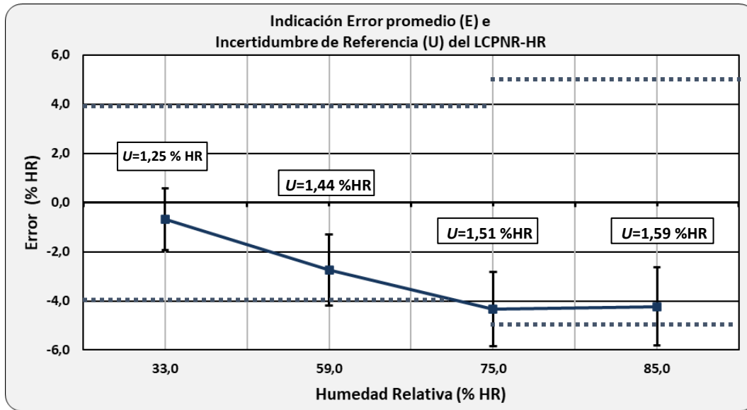
Gráfico 3. Error promedio, E , e incertidumbre del laboratorio de referencia, U ( k=2 , 95%), con consideración adicional por deriva del patrón viajero . (Las líneas de puntos corresponden a la exactitud del instrumento).
