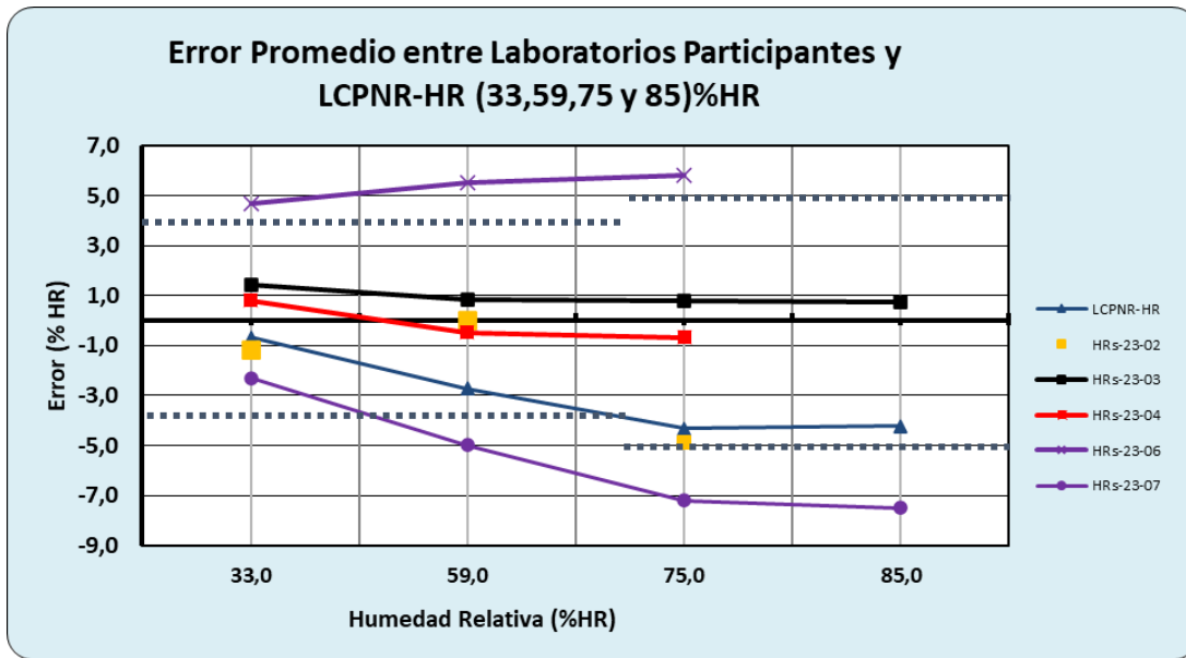
Gráfico 5. Error promedio de laboratorios participantes. (Las líneas de puntos corresponden a la exactitud del instrumento).
